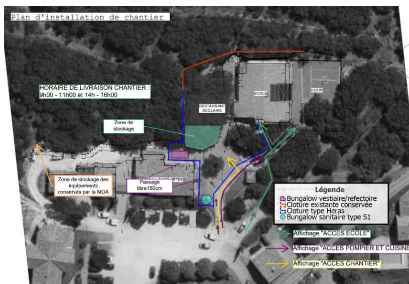
Plan d'installation de Chantier
